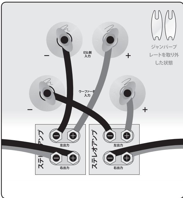
水平バイアンプ接続、片チャンネル
