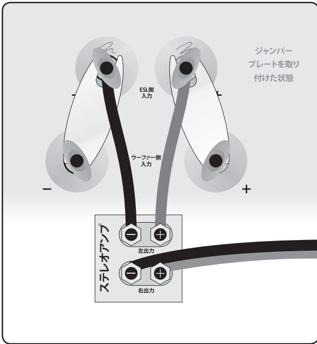
シングルワイヤー接続、片チャンネル
