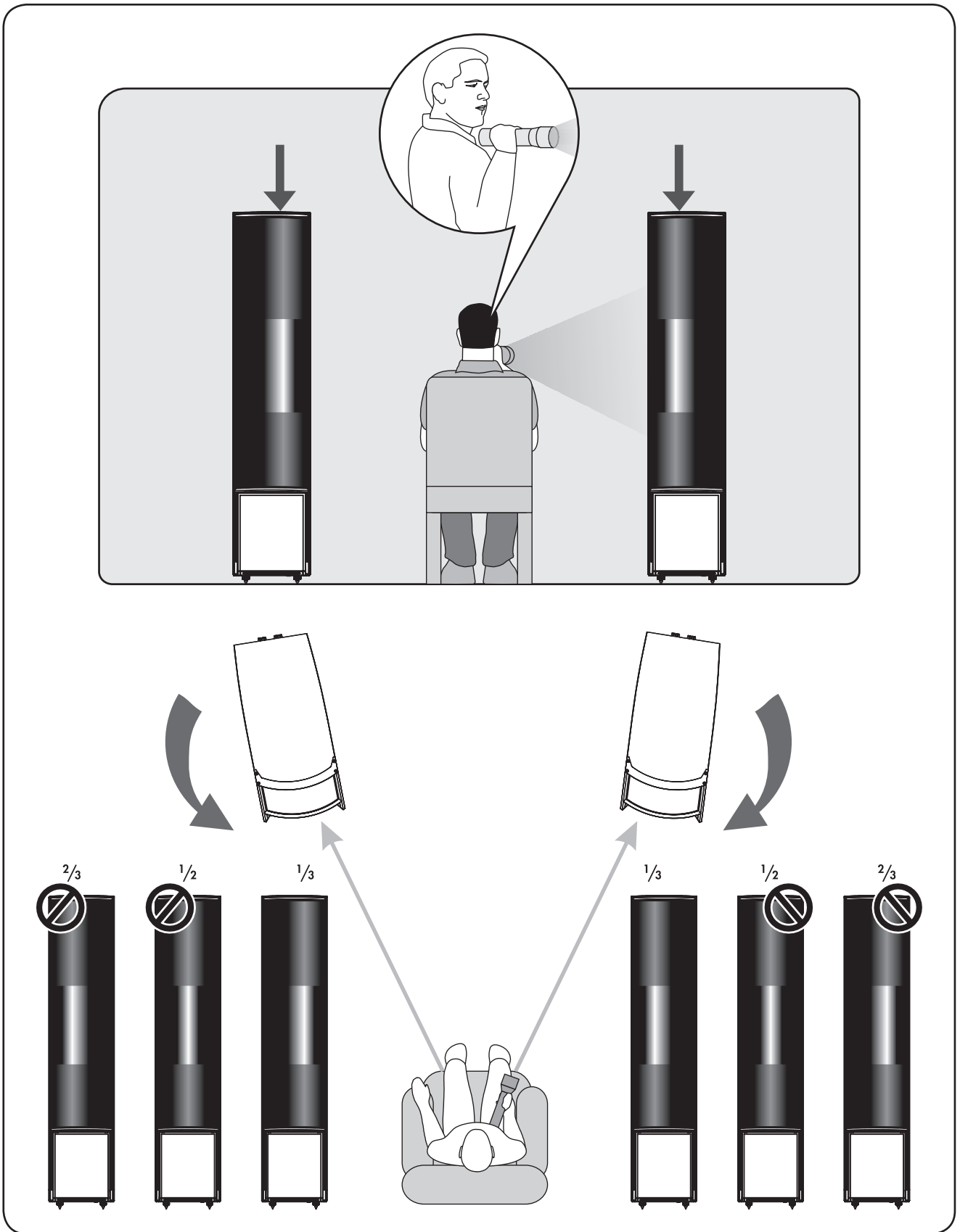
懐中電灯を使ったトウイン角度の設定
