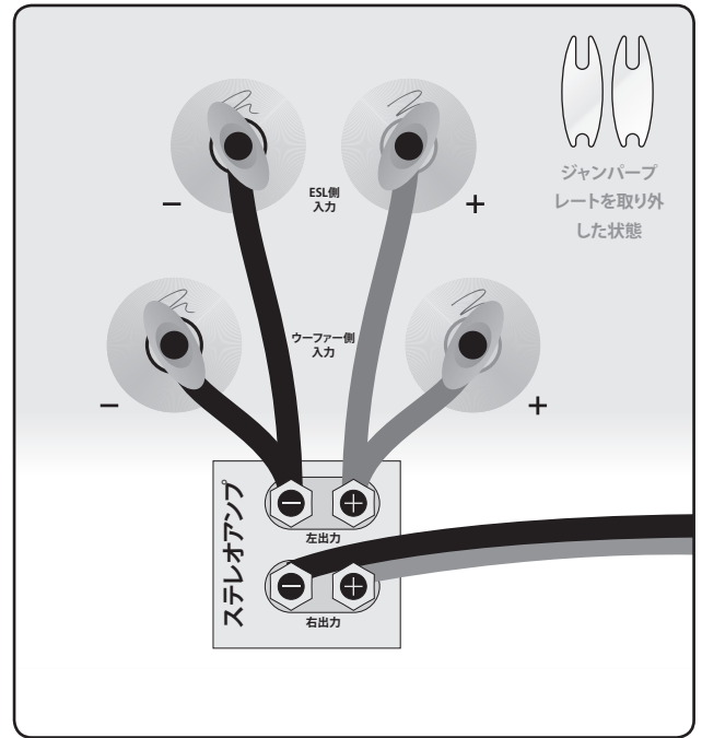
バイワイヤー接続、片チャンネル
