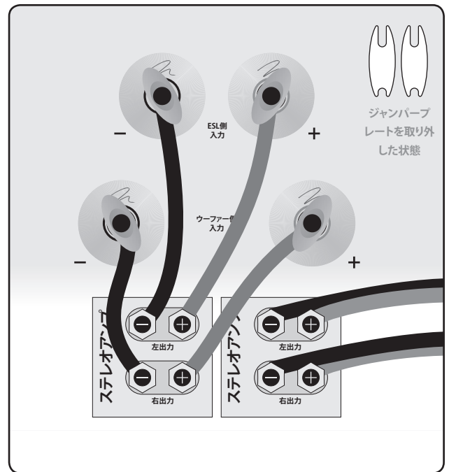
垂直バイアンプ接続、片チャンネル
